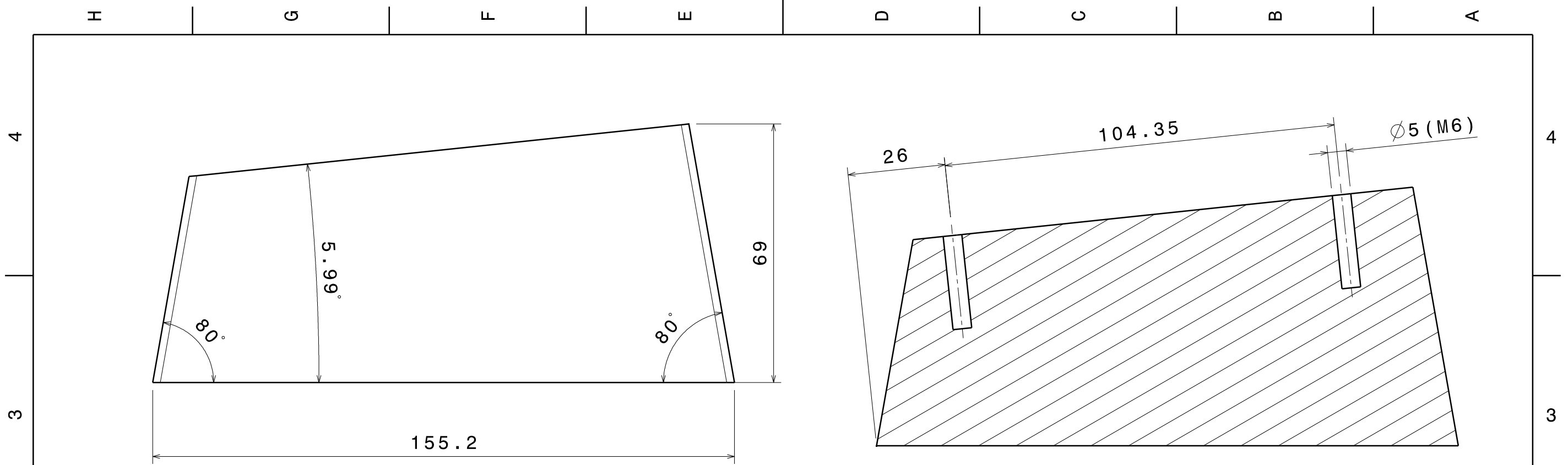
Section view A-A Scale: 1:1
